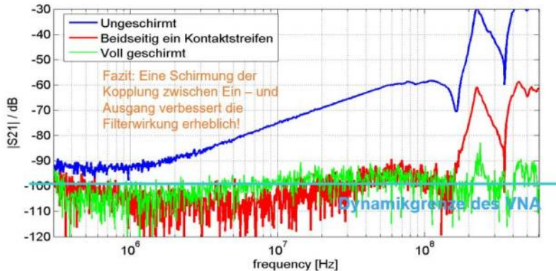
Kontaktstreifen
