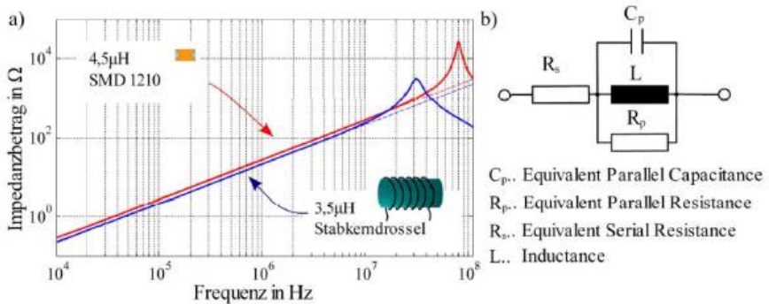
a) Impedanz verschiedener Spulenformen, b) HF-Ersatzschalbild.
