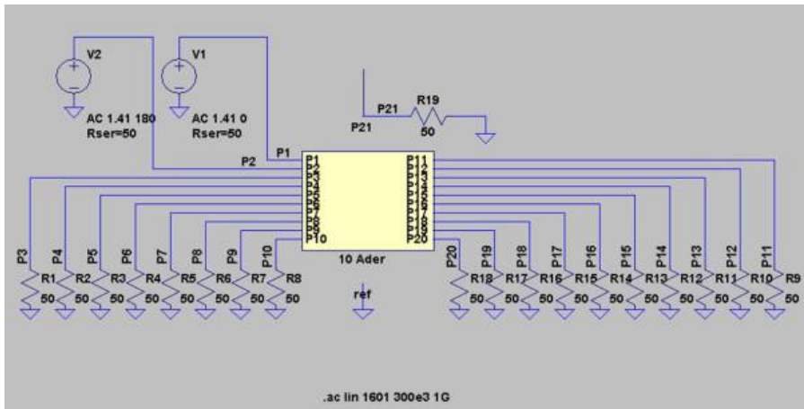
Abbildung: Beispiel zur Analyse in SPICE, dargestellt: Anregung Leiter 1 und Leiter 2 mit Gegentakt
